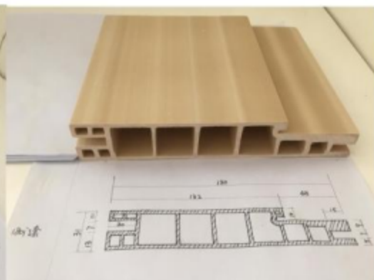
18031门框 18031 Door Frame
