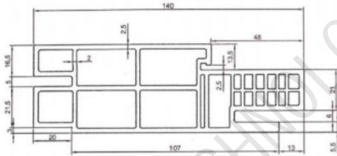
12046外贸门框 12046 Door Frame
