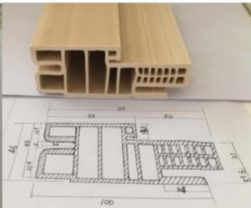
10046外贸门框 10046 Door Frame
