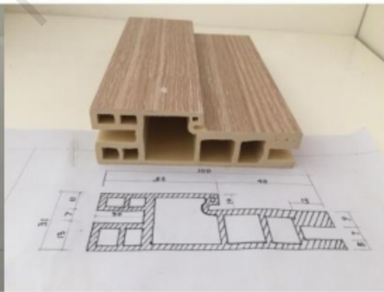
10031门框 10031 Door Frame
