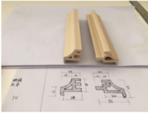
2332玻璃压条(2332 Glass beading)
