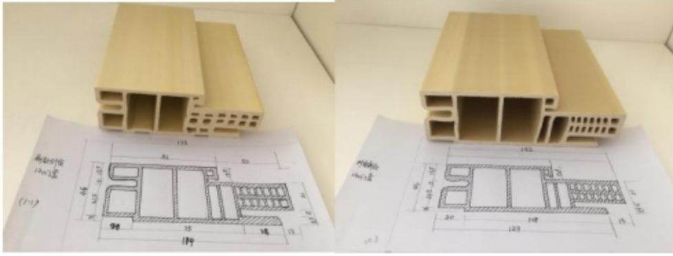
12046外贸门框 12046 Door Frame
